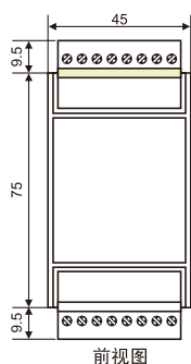
前视图
